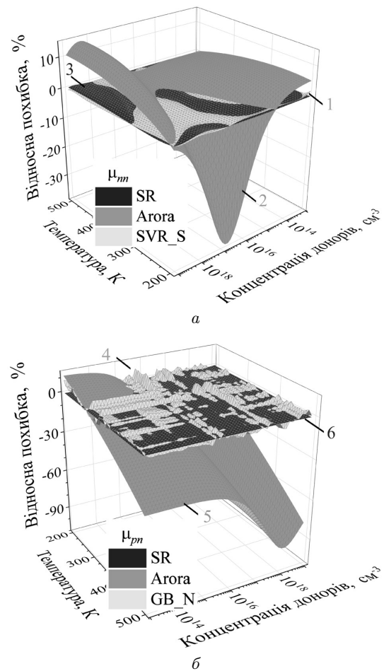
Рис. 4. Температурні й концентраційні залежності помилок розрахунків рухливості основних (а) і неосновних (б) носіїв за допомогою різних моделей відповідно до теорії Клаассена. Модель: SVR_S (поверхня 1), Arora (2, 5), SR (3, 6), GB_N (4)
